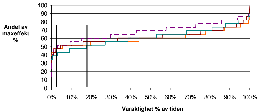
Figur 7. Procentuellt utnyttjande av huvudsäkringen sorterade i storleksordning. Exempel framgår av texten ovan.
