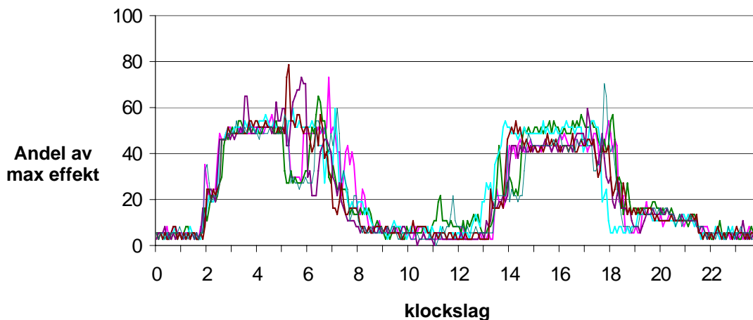
Figur 5. Medeleffekt för 5 minuter under sex dagar i april 2005 på gård B.
