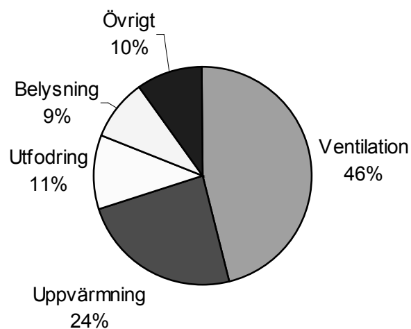
Figur 1) Energiförbrukare i en slaktgrisproduktion, % (JBT, SLU Rapport 145, 2007).
